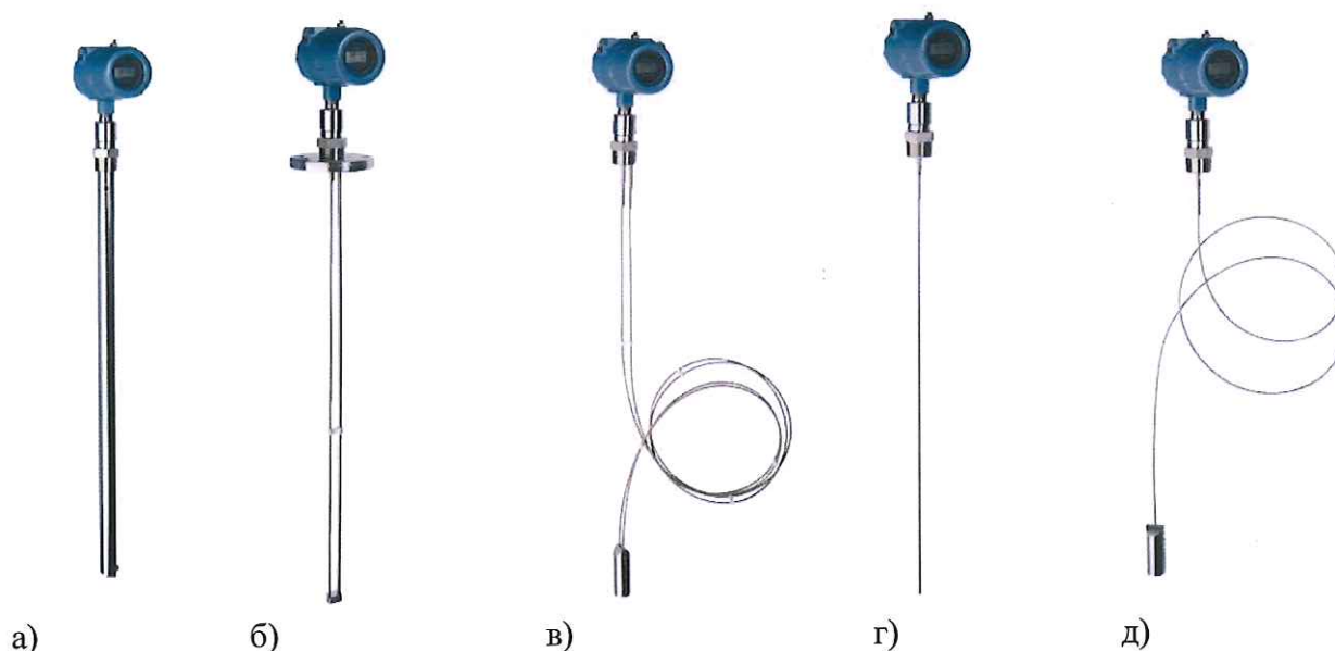
Рисунок 1 - Общий вид уровнемеров 3300 с различными типами волноводов (зондов): а) коаксиальный, б) жесткий двойной, в) гибкий двойной с грузом, г) жесткий одинарный, д) гибкий одинарный с грузом
