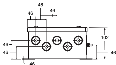
Вид спереди
