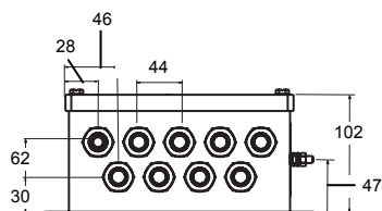
Вид спереди
