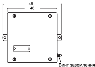
Вид спереди
