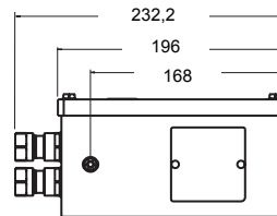
Вид сбоку
